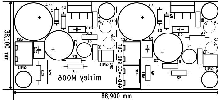
Mini Wzmacniacz 2x15W Pobrane z http://mirley.net
