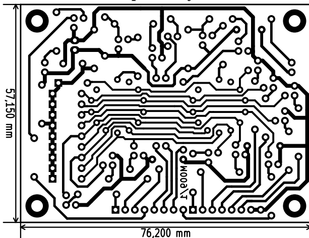
Prosty zegar Nixie z termometrem Pobrane z http://mirley.net
